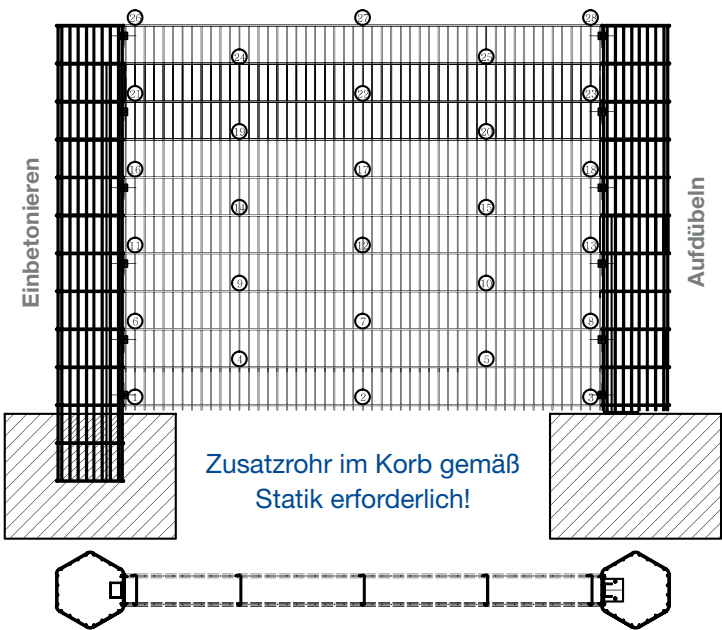
Technische Zeichnung
